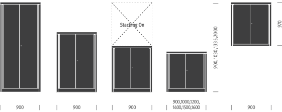
CK2 Sliding Door Cabinet
