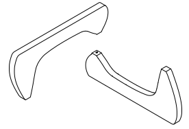
Leg (Qty: 2)
